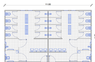
PLANTA BAIXA
