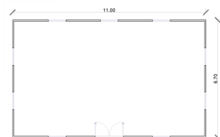
PLANTA BAIXA
